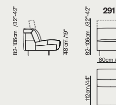
1 místný sedací díl bez područky
